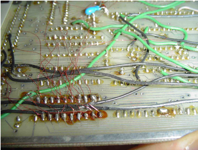
Abbildung: Fehlerbeseitigung eines Floppycontrollers
